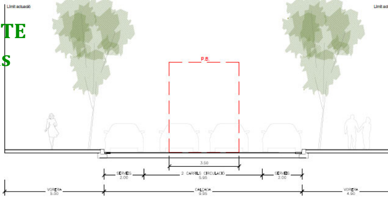
ST2 | ST3 C/ DE BISCAIA ESTAT ACTUAL escala 1:100
