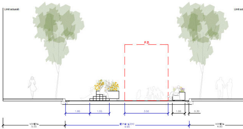
ST2 C/ DE BISCAIA PROPÒSITA escala 1:100
