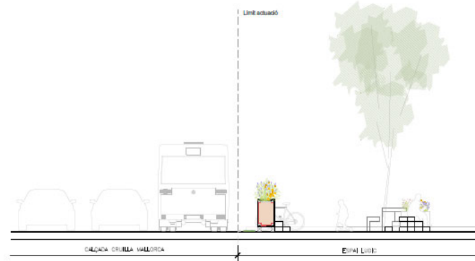
ST4 C/ DE BISCAIA PROPOSTA ESCALA 1:100
