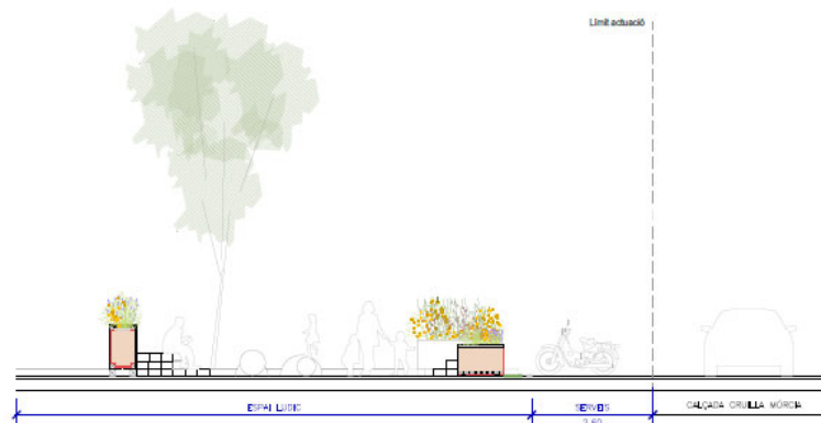
ST5 C/ DE BISCAIA PROPOSTA ESCALA 1:100
