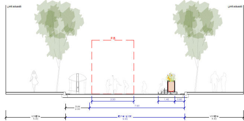
ST3 C/ DE BISCAIA PROPÒSITA escala 1:100
