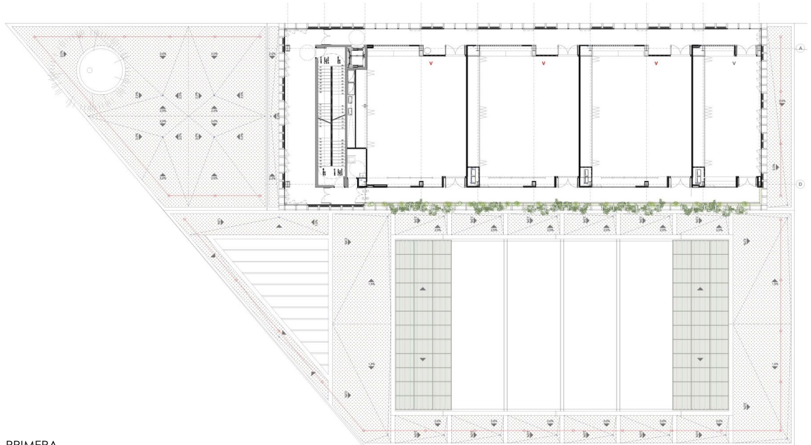
PLANTA PRIMERA
