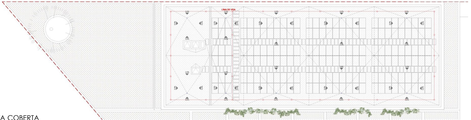
PLANTA COBERTA
