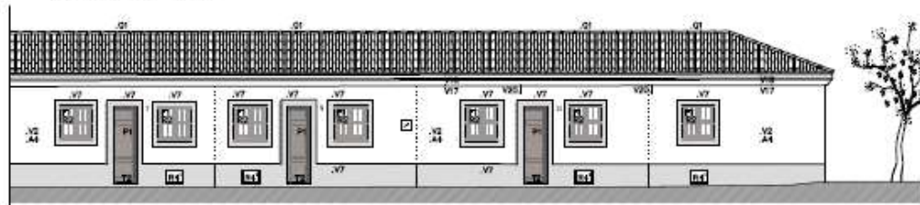
ALÇAT C/ BELLMUNT – SECTOR A E 1:100
