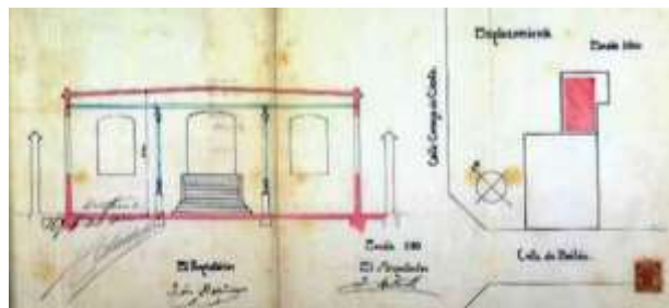
1913. Secció del projecte de Jeroni Martorell. Amb estructura de pilars de fosa..
