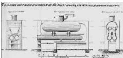
ACMB, Núm. Exp. 1.919, any 1853, Plànol de la caldera de vapor dels senyors "Rosés i Companyia" al carrer de Ramon Berenguer el Vell núm. 1.
