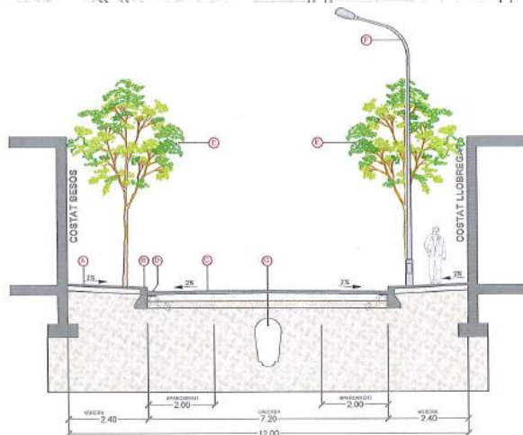
SECCIÓ A-A' i B-B' ACTUAL 1/100
