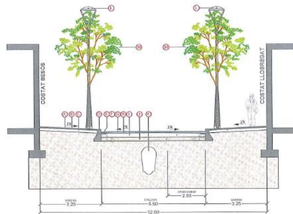
SECCIÓ A-A' i B-B' PROPOSTA 1/100
