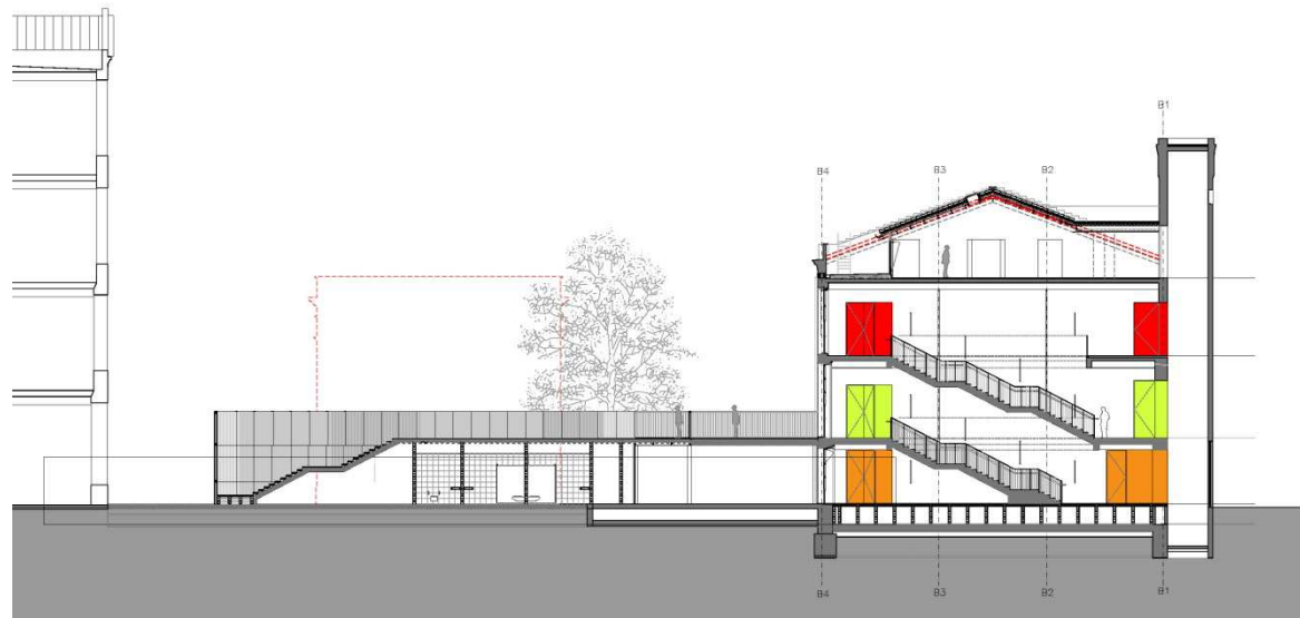
Secció transversal
