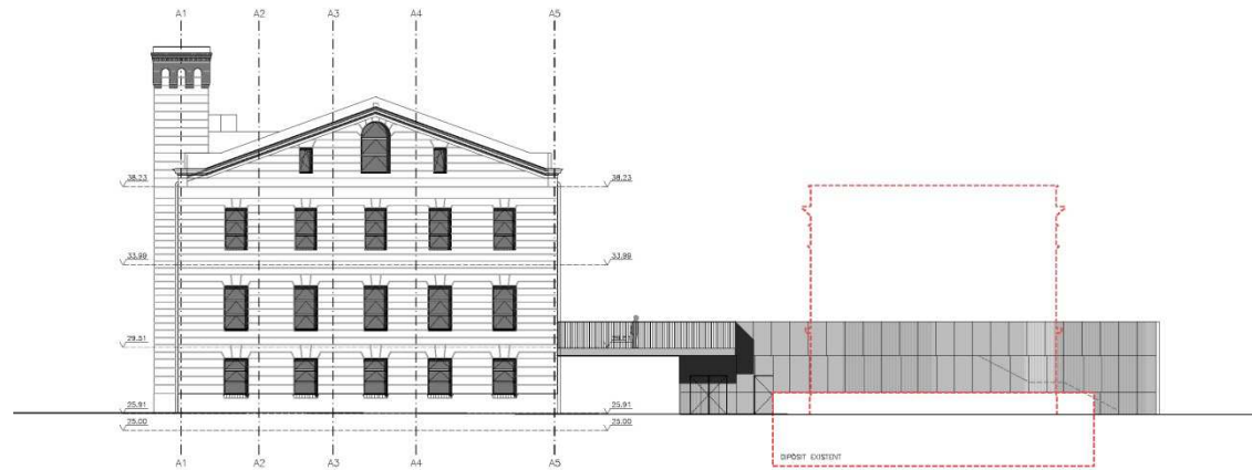
Alçat oest
