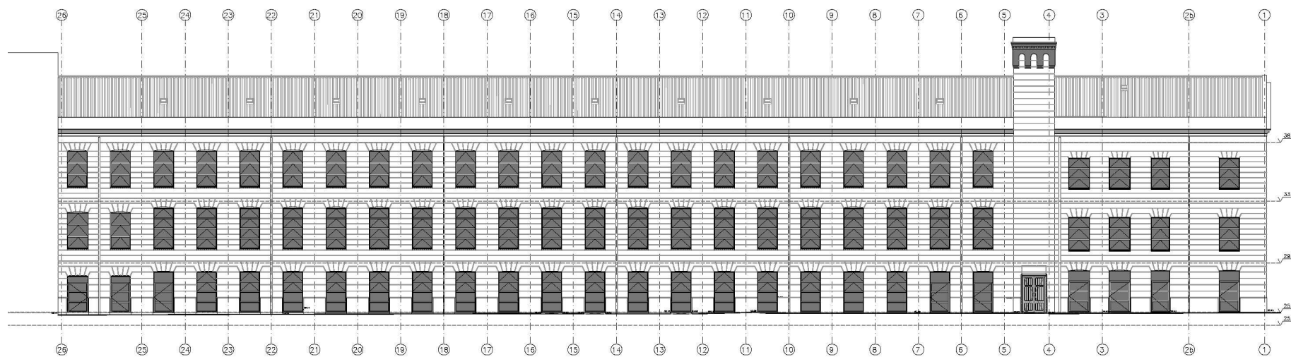
Alçat nord
