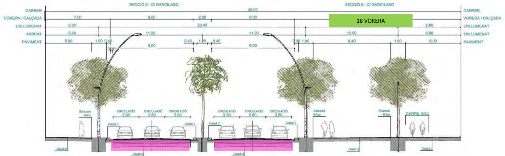
SECCIÓ PROJECTE D'URBANITZACIÓ APROVAT 2012 SECCIÓ 6 - C/ GARCILASO
