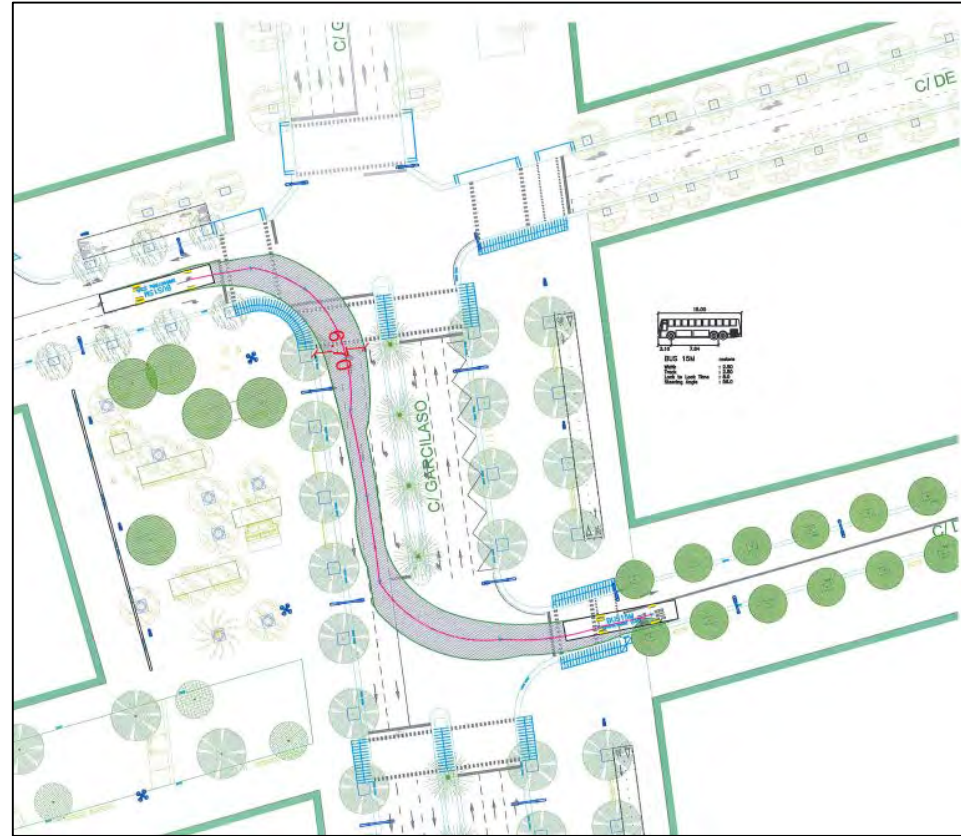
GIR DES DE CARRIL ESQUERRE ( GRAN DE LA SAGRERA)
