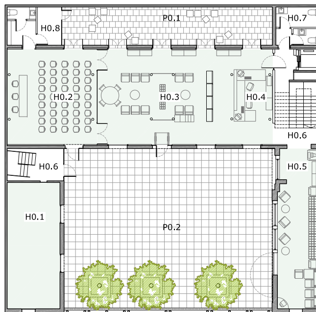
PLANTA ACCÉS
