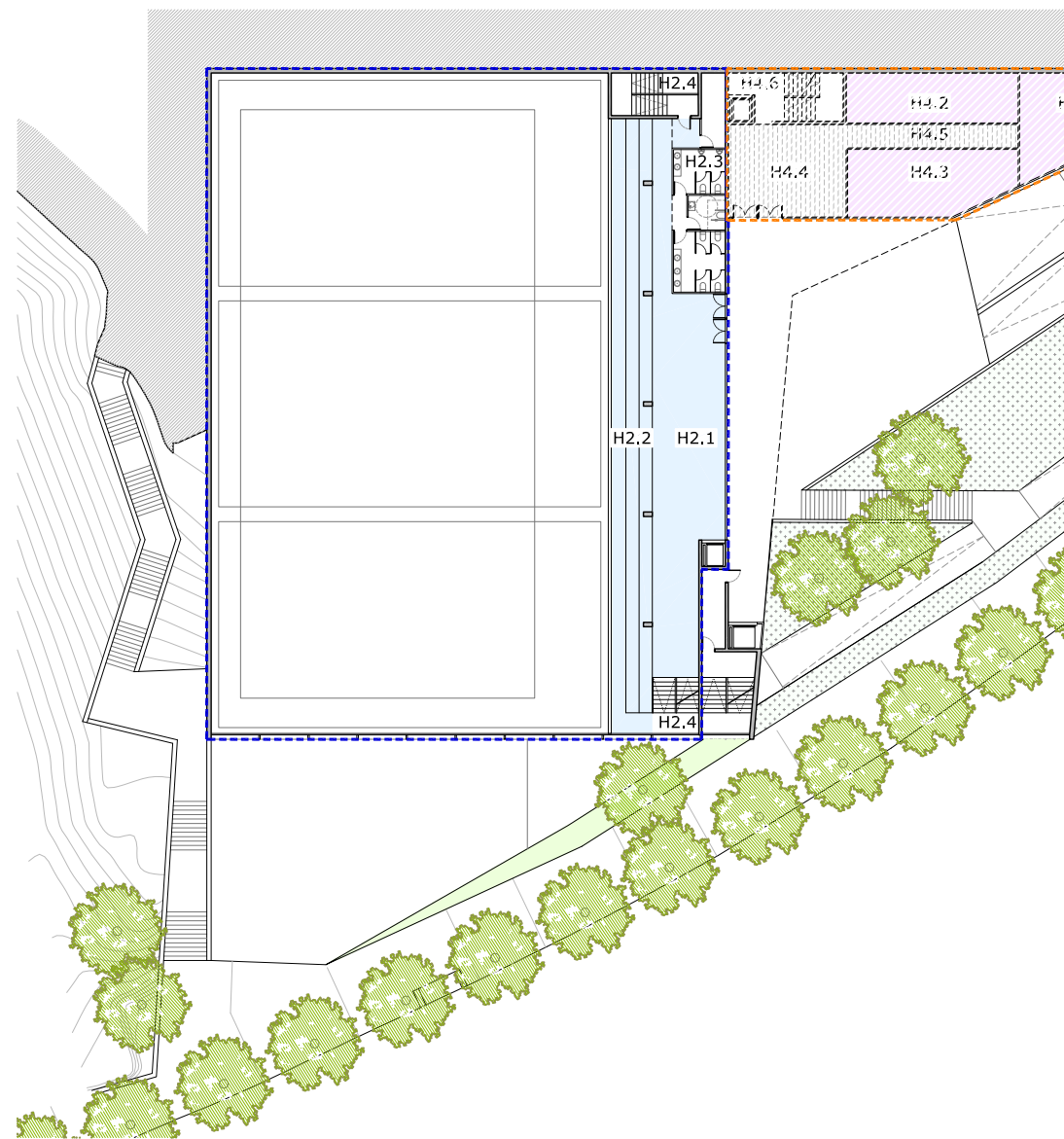
NIVELL 3 COTA +46,00
