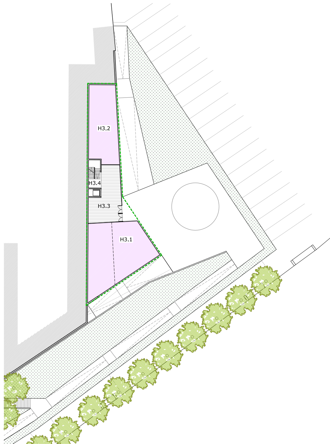
NIVELL 3 COTA +44,00
