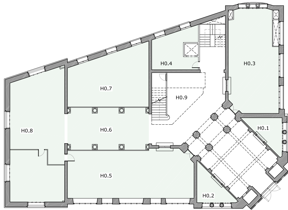
PLANTA BAIXA
