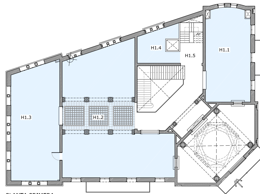
PLANTA PRIMERA
