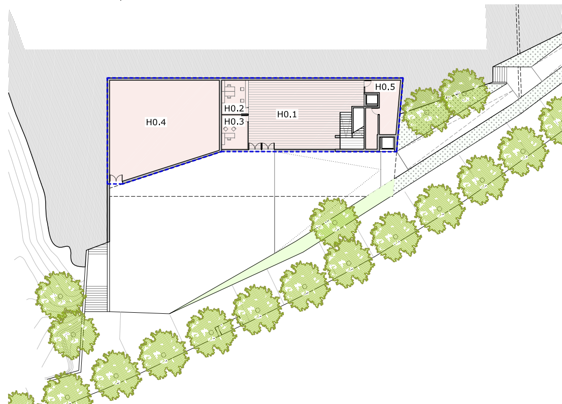
NIVELL 0 COTA +37,50
