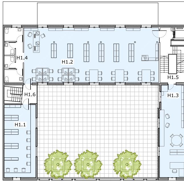
PLANTA PRIMERA
